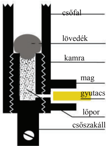
Delvigne csőfar
