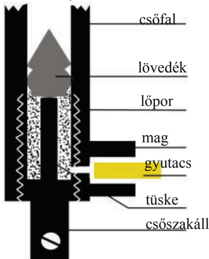
Thovenien csőfar
